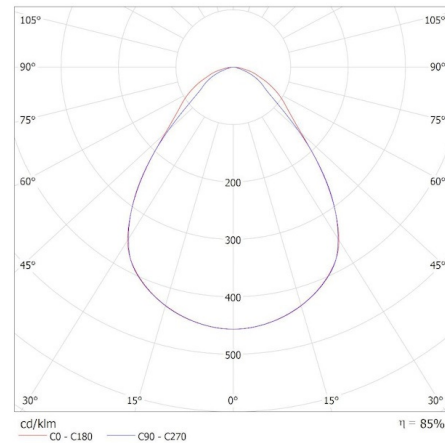
KANLUX S.A. (kat 37274) BLINGO 28-35W 6262 CCT 4000K / Krzywa rozsyłu światła (biegunowo)
